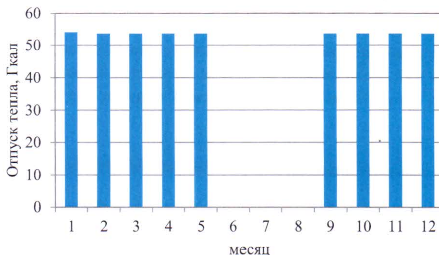
Рис. 3 – Оптимальный температурный график отпуска тепловой энергии для котельной с. Новоникольское
