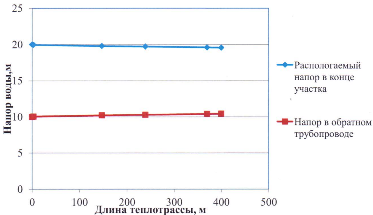
Рис. 5 – Пьезометрический график тепловой сети котельной с. Новоникольское
