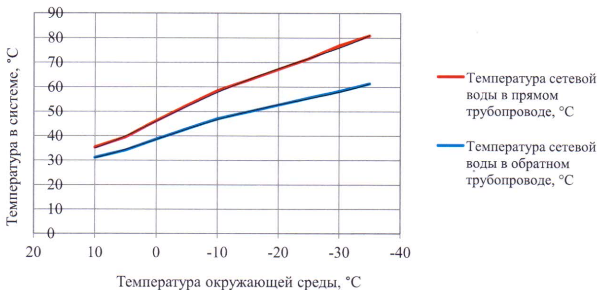
Рис. 4 – График изменения температур теплоносителя
